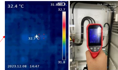
ตรวจสอบความร้อนฟิวส์ MCCB 32.7 °C
