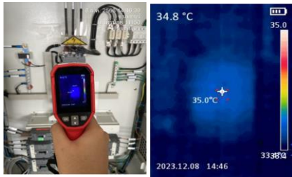
ตรวจสอบความร้อนMCCB 35.0 °C
